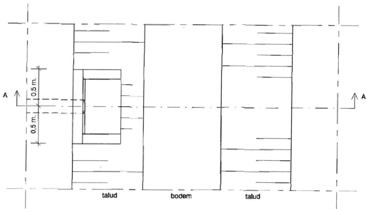
Bovenaanzicht
