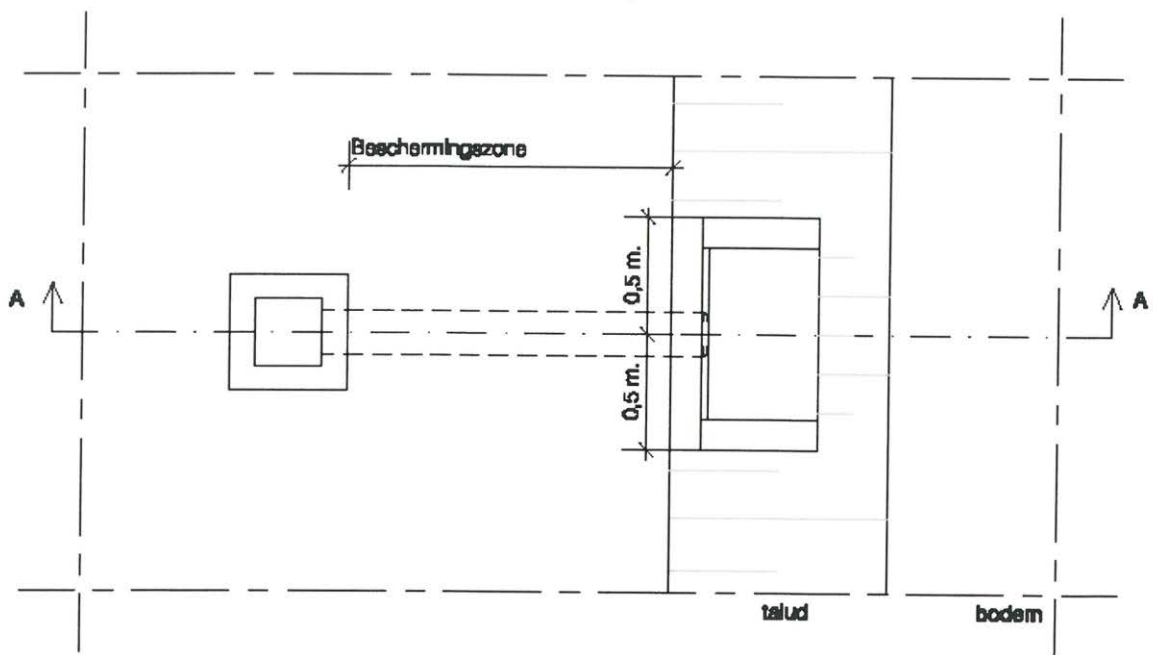
Bovenaanzicht
