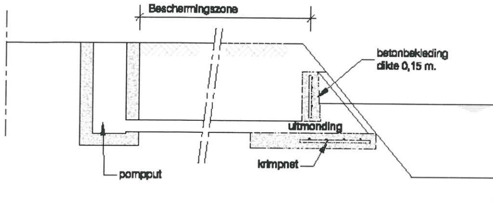
Dwarsdoorsnede A-A
