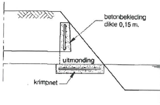
Dwarsdoorsnede A-A
